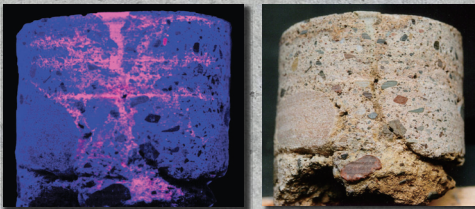
【UVライトをあてての実験】 ピンク色の部分がコンクリートへの浸透を示しています。
